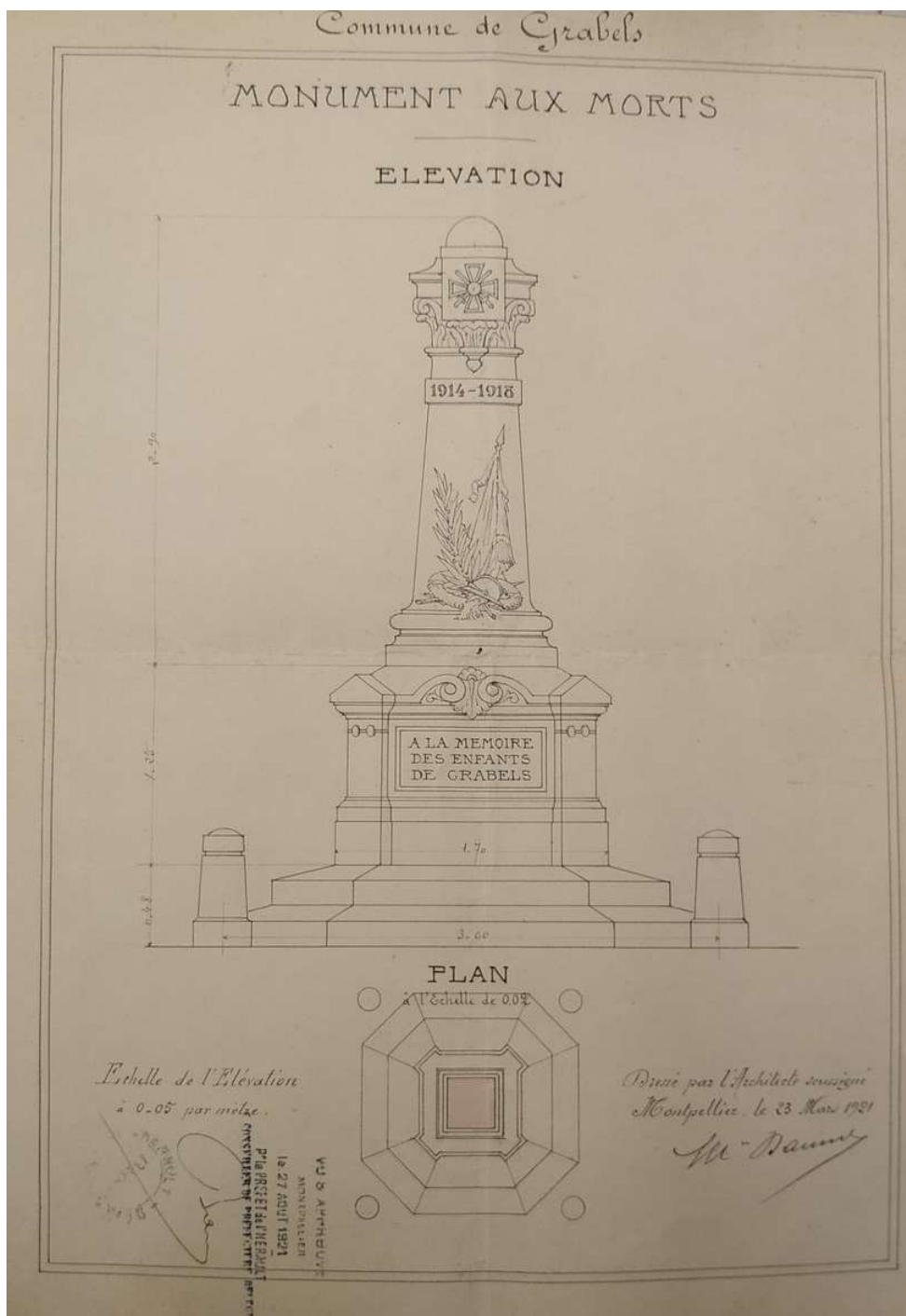
Plan et élévation du monument aux Morts, 1921 (1M5)
